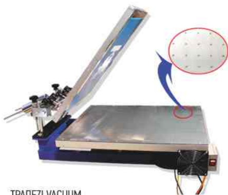
ΤΡΑΠΕΖΙ VACUUM για διάφορους πάγκους εργασίας 50 x 60 cm
