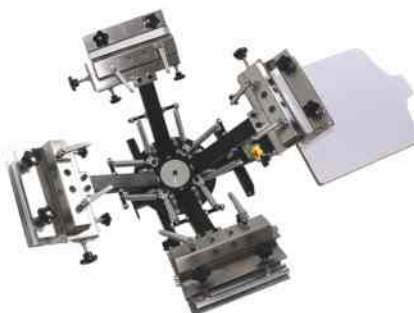
ΜΗΧΑΝΙΣΜΟΣ ΜΕΤΑΞΟΤΥΠΙΑΣ 4 ΧΡΩΜΑΤΑ ΜΕ MICRO REGISTRATION Χειροκίνητη μηχανή μεταξοτυπίας χωρίς πόδια με 4 χρώματα / 4 σταθμούς για μπλούζες με σύστημα micro registration και παλέτες αλουμινίου. Μέγιστη διάσταση τελάρου 50 x 60 cm
